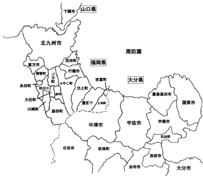
【図3】 豊前南部地域とその周辺図 (筆者作成)
