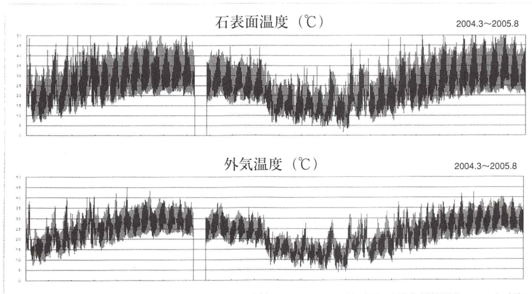
Fig. 5 石表面温度と外気温度の比較
