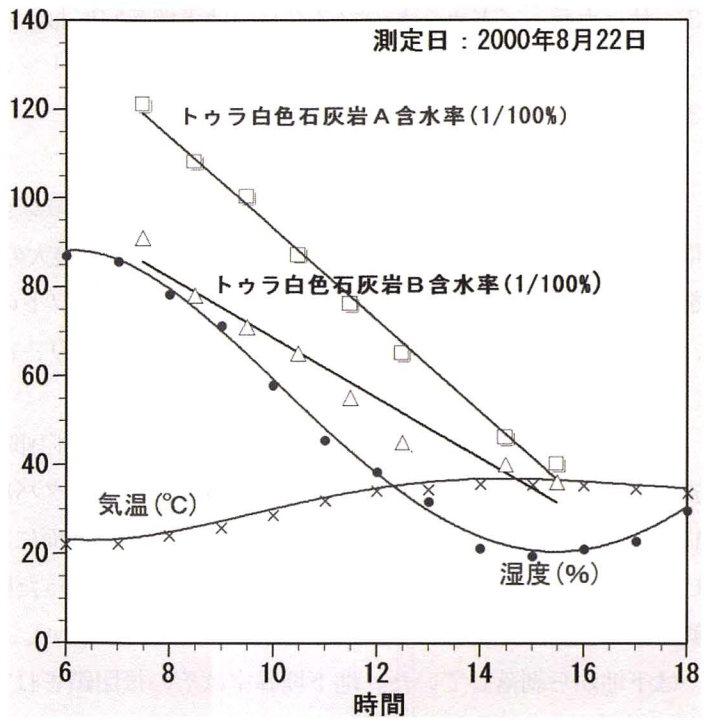
Fig. 7 1日の温度、湿度変化と岩石表面含水率の関係
