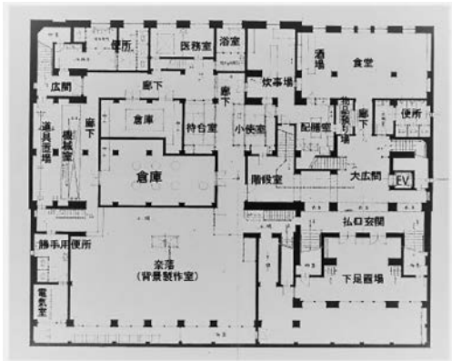
図 2-5 先斗町歌舞練場 地階平面図
