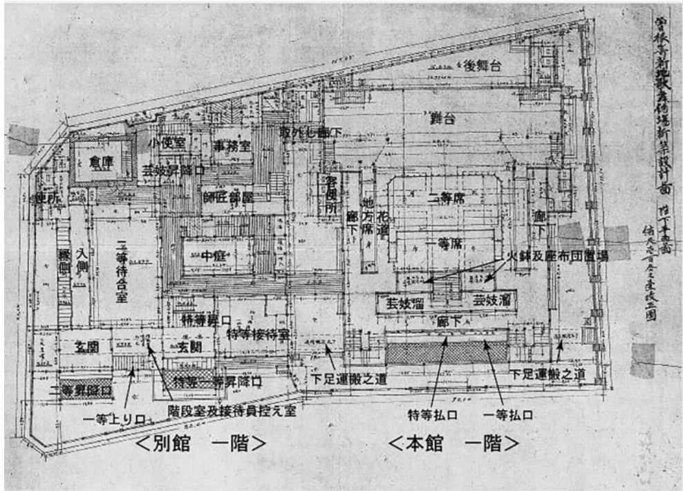
圖 1-1 北陽演舞場 1階平面圖
