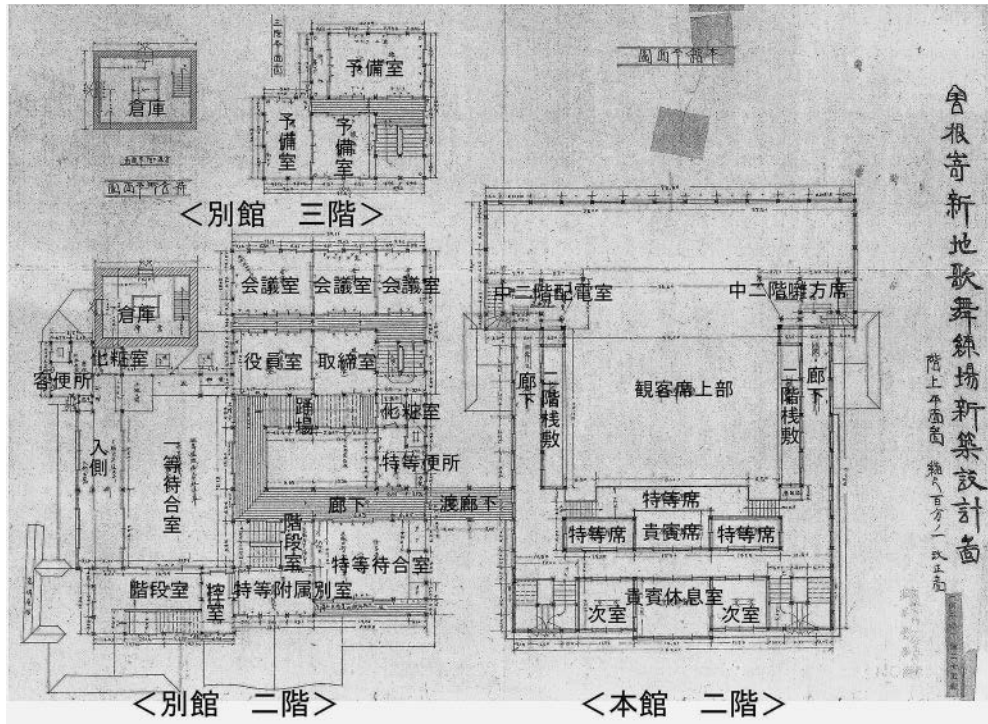
圖 1-2 北陽演舞場 2階・一部3階平面圖
