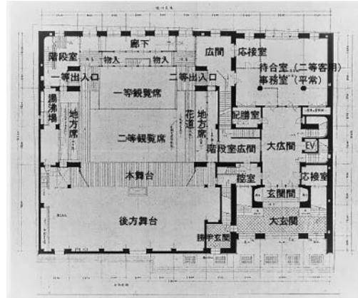
図 2-1 先斗町歌舞練場 1階平面図 (左が北、以下同様)
