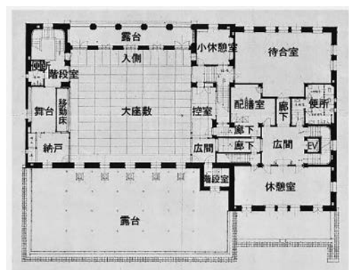
図 2-3 先斗町歌舞練場 3階平面図
