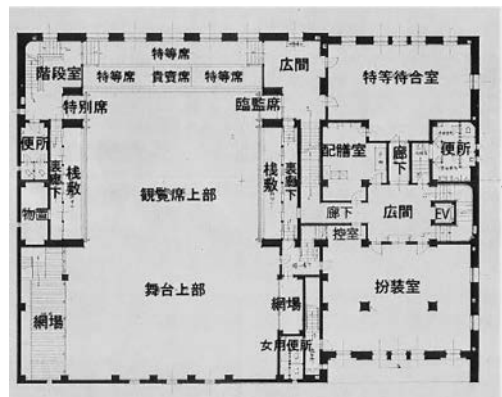
図 2-2 先斗町歌舞練場 2階平面図
