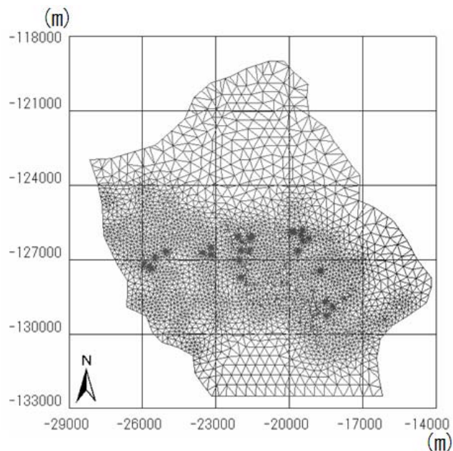
図 22 平面メッシュ図
