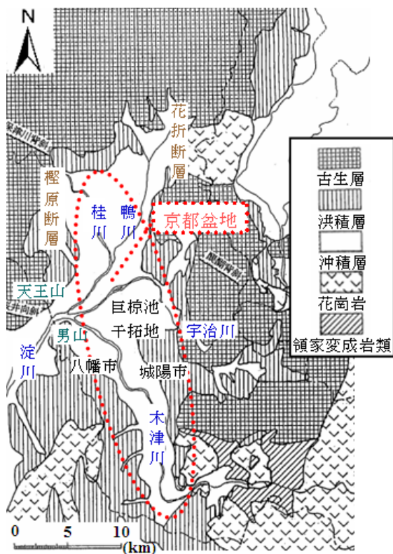
図 2 京都盆地の地質分布 (文献8)に加筆
