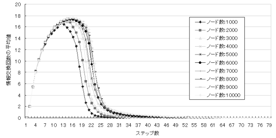
図 19 ステップごとの情報交換回数の平均値 (一様分布)
