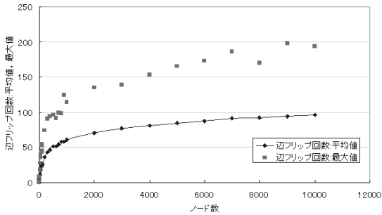
図 16 ノード数に対する辺フリップ回数の平均値, 最大値 (一様分布)
