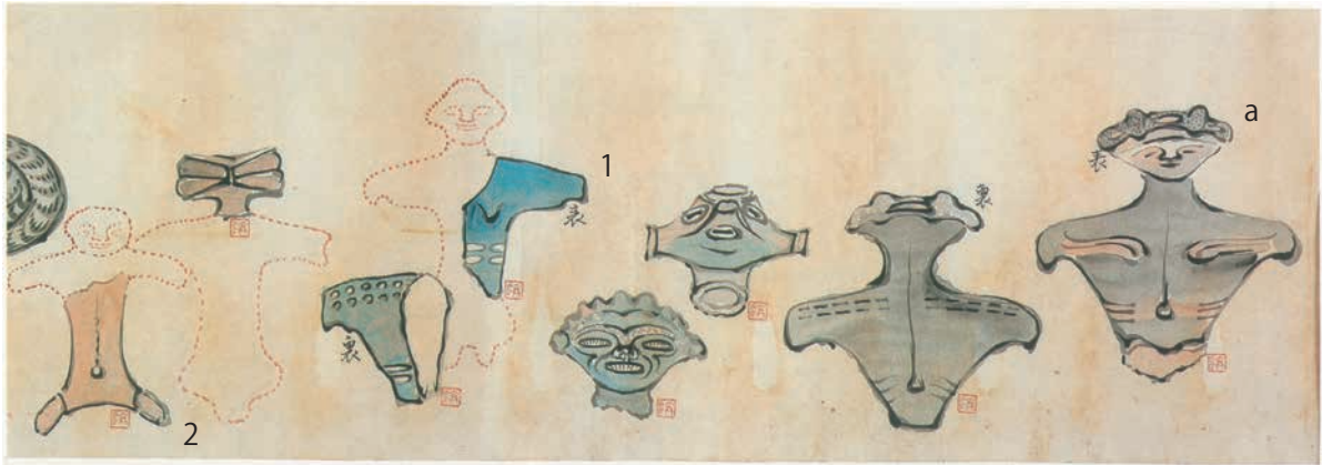
第2図 陸奥全国神代石井古陶之図にみえる本山コレクションの土偶
