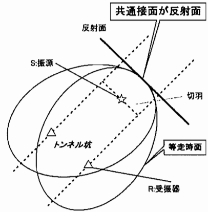
図-3 柵面群の共通接面による反射面のイメージング
