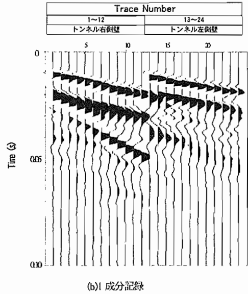
図-7 現場記録
