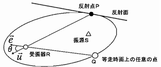
図-3 柵面群の共通接面による反射面のイメージング
