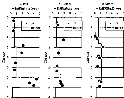
図-8 一軸圧縮強度の深度方向分布
