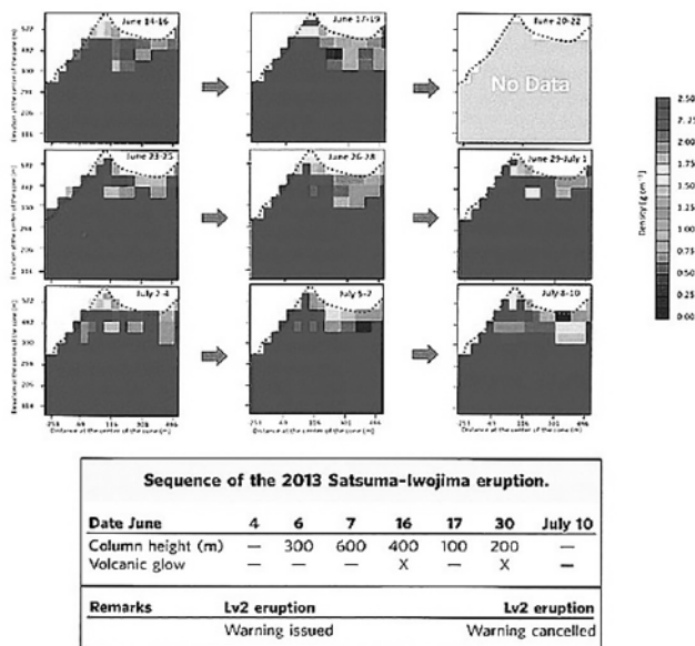
図3 オリジナルのミュオグラフィ画像 [2] Fig. 3. Original muography images. [2]
