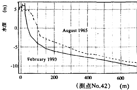
図-9 海浜断面の比較例
