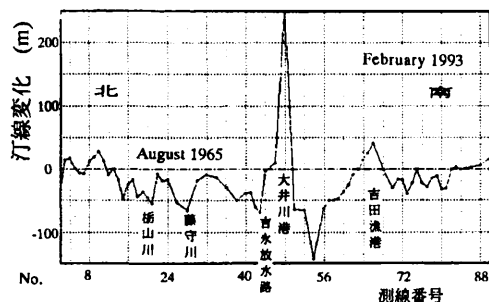
図-7 汀線変化図
