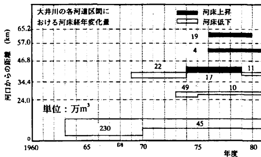
図-4 河床の経年変化量
