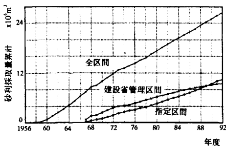
図-5 累計砂利採取量
